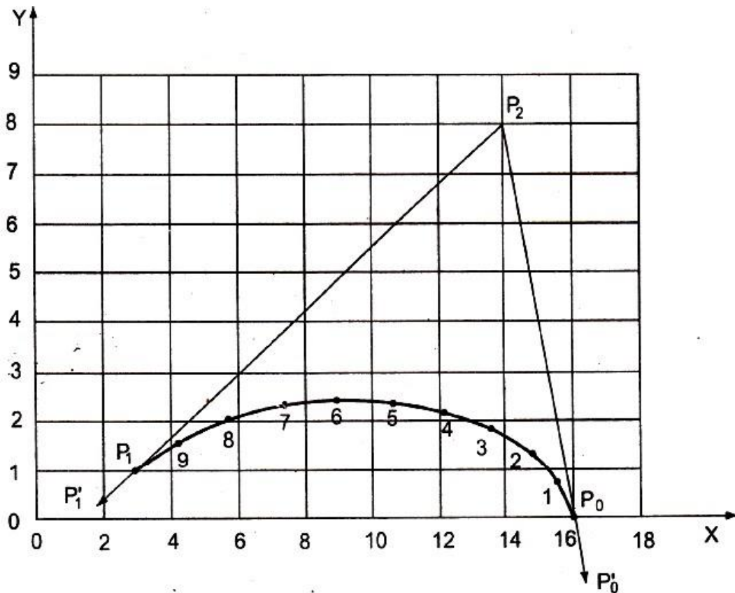
Fig. 2.13
